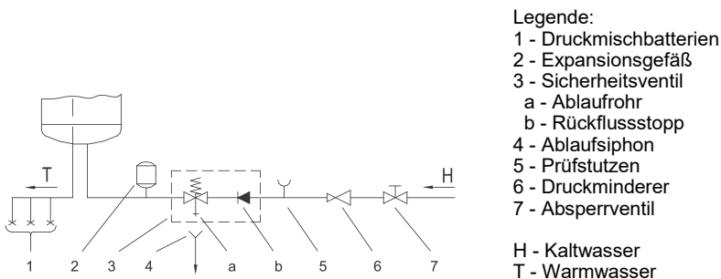
Abb. 2: Geschlossenes System (druckfestes System)
