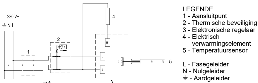
Fig. 4: Elektrische installatie
