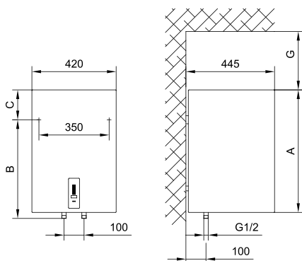
Fig. 1: Verticale installatie tegen een muur
