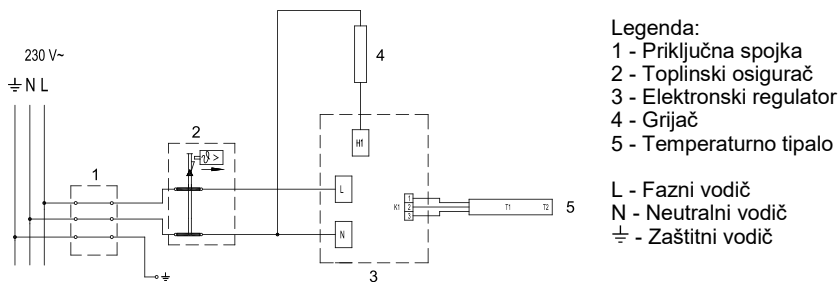
Sl. 4: Električna spojna shema
