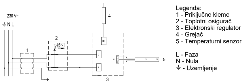
Sl. 4: Šema povezivanja električnih provodnika
