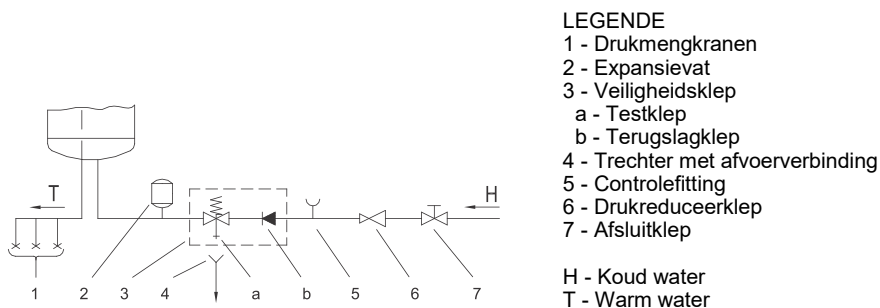
Fig. 2: Gesloten (druk)systeem
