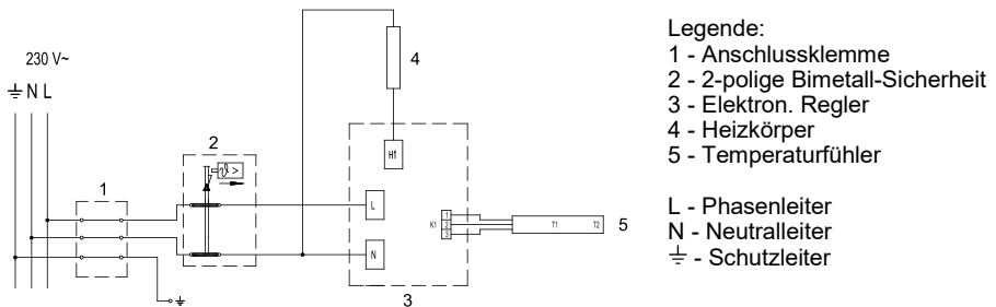
Abb. 4: Elektroschaltbild
