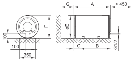
SI. 2: Vodoravno montiranje na pod
