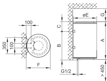
Fig. 1: Verticale installatie tegen een muur
