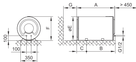
SI. 2: Ležeča namestitev na tla
