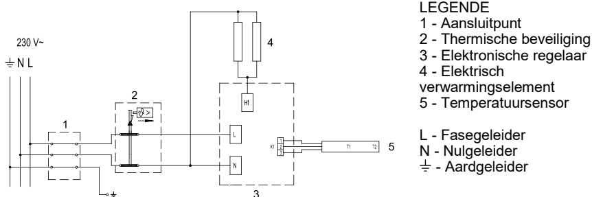
Fig. 5: Elektrische installatie
