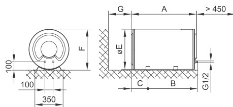
Abb. 2: Waagrechte Montage am Boden
