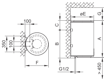
SI. 1: Vertikalno montiranje na zid
