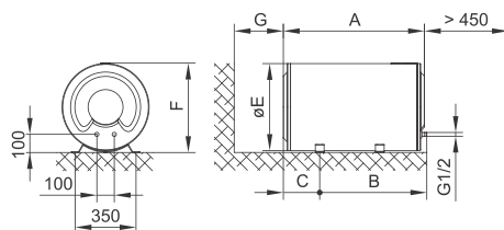
Fig. 2: Horizontale installatie op de vloer
