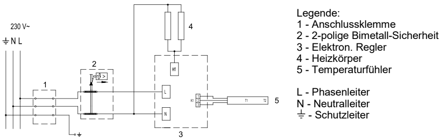
Abb. 5: Elektroschaltbild
