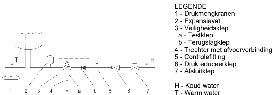
Fig. 3: Gesloten (druk) systeem
