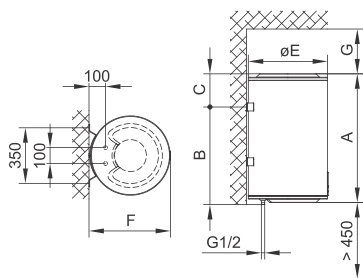
Abb. 1: Senkrechte Montage an die Wand
